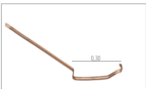
Tirante K7 Sviluppo 415
